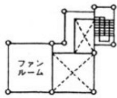
中地1階平面図
